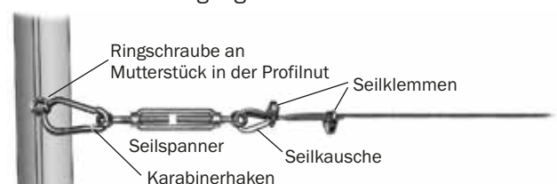
untere Netzbefestigung:
